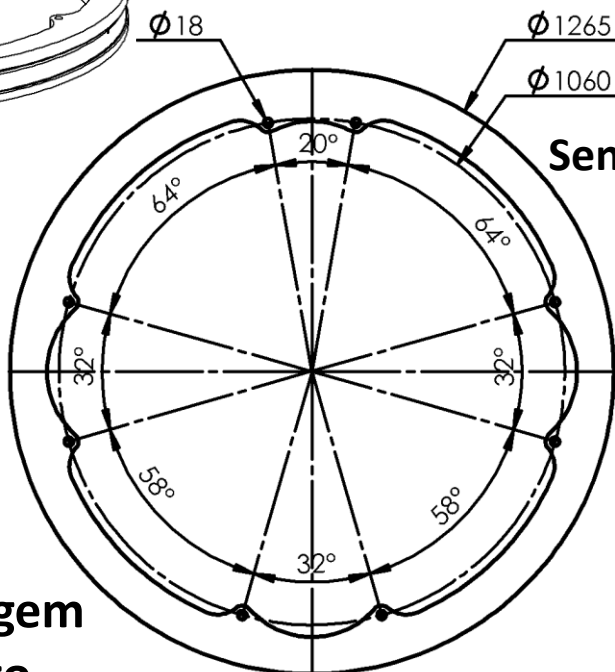
Anel inferior
